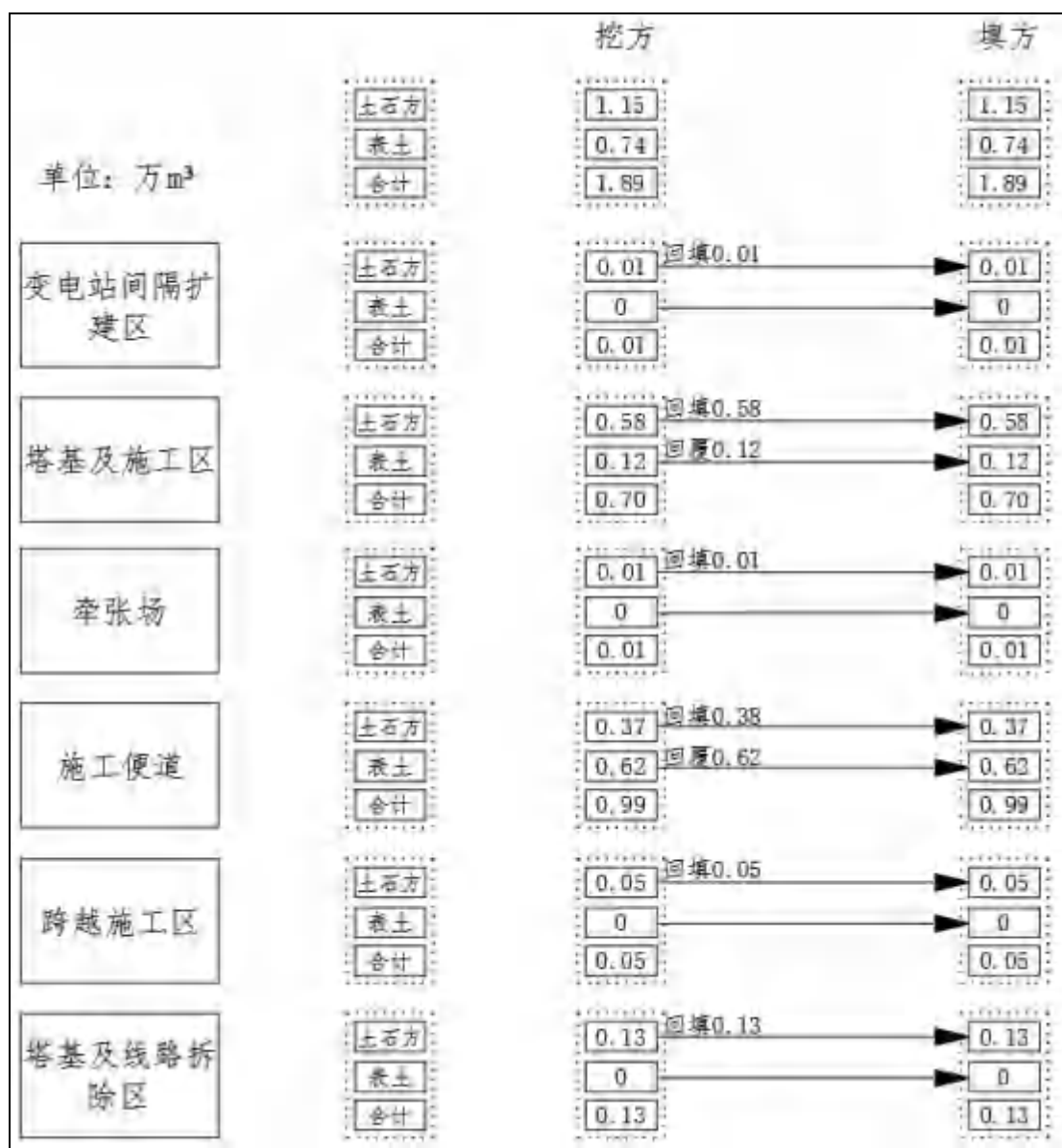
图 2-4 总土石方流向框图
